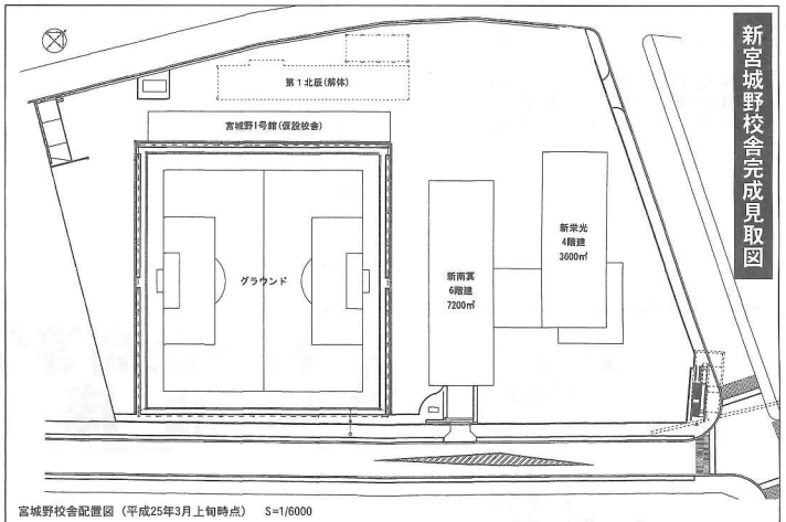
宮城野校舎配置図 (平成25年3月上旬時点) S=1/6000
