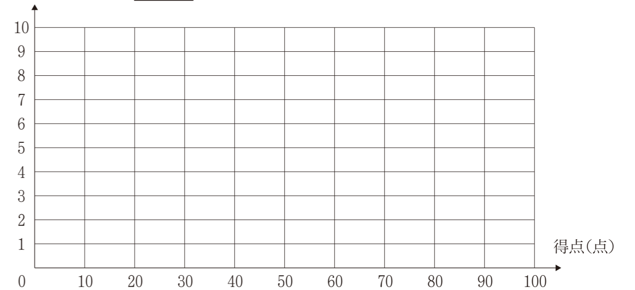
児童の数(人) 第3問 (3) ヒストグラム (柱状グラフ)
